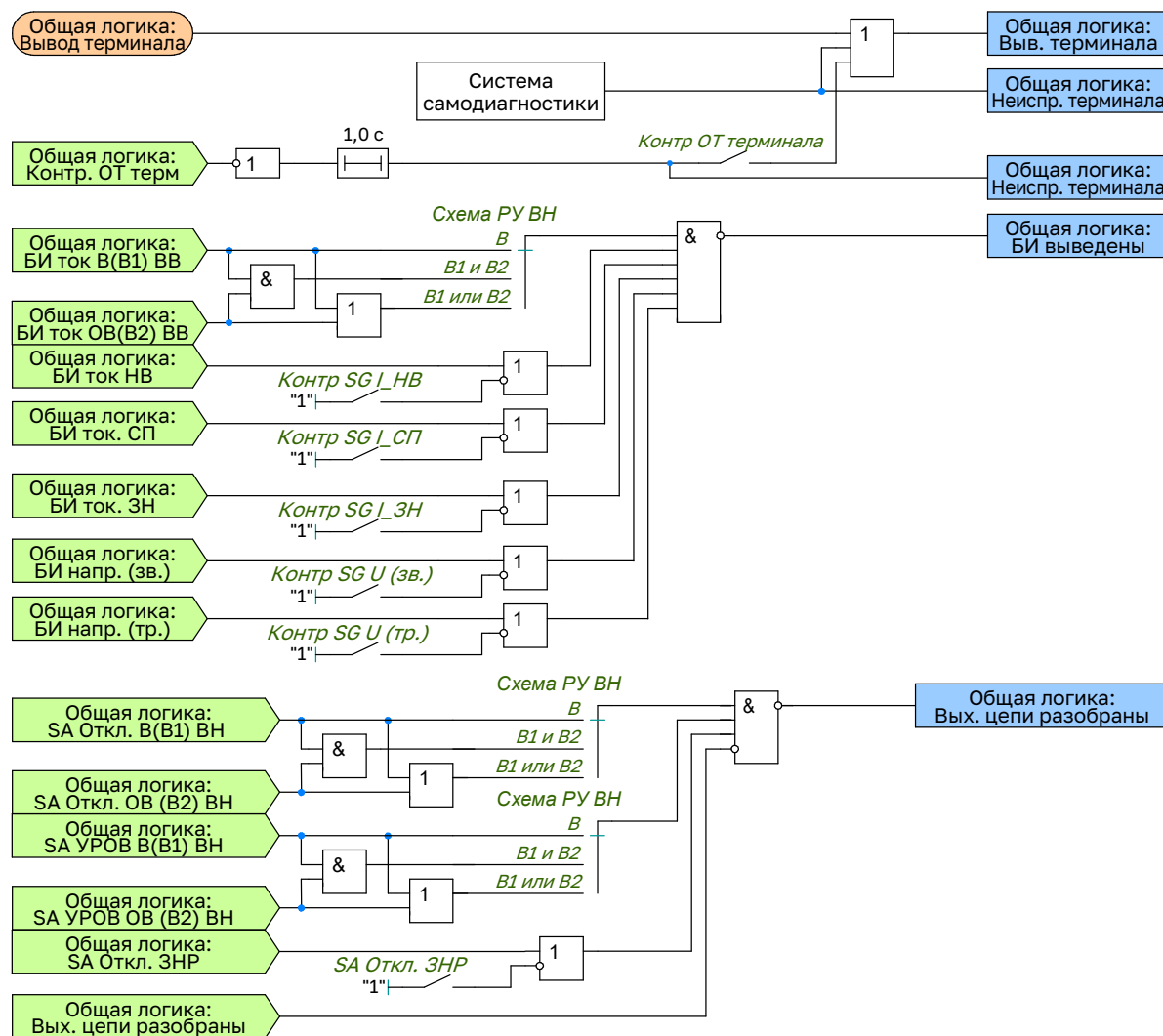
Рисунок 2.36 – Функциональная схема общей логики
