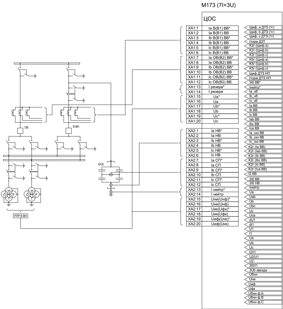
Рисунок Б.1 – Вариант подключения аналоговых цепей ТТ и ТН к устройству
