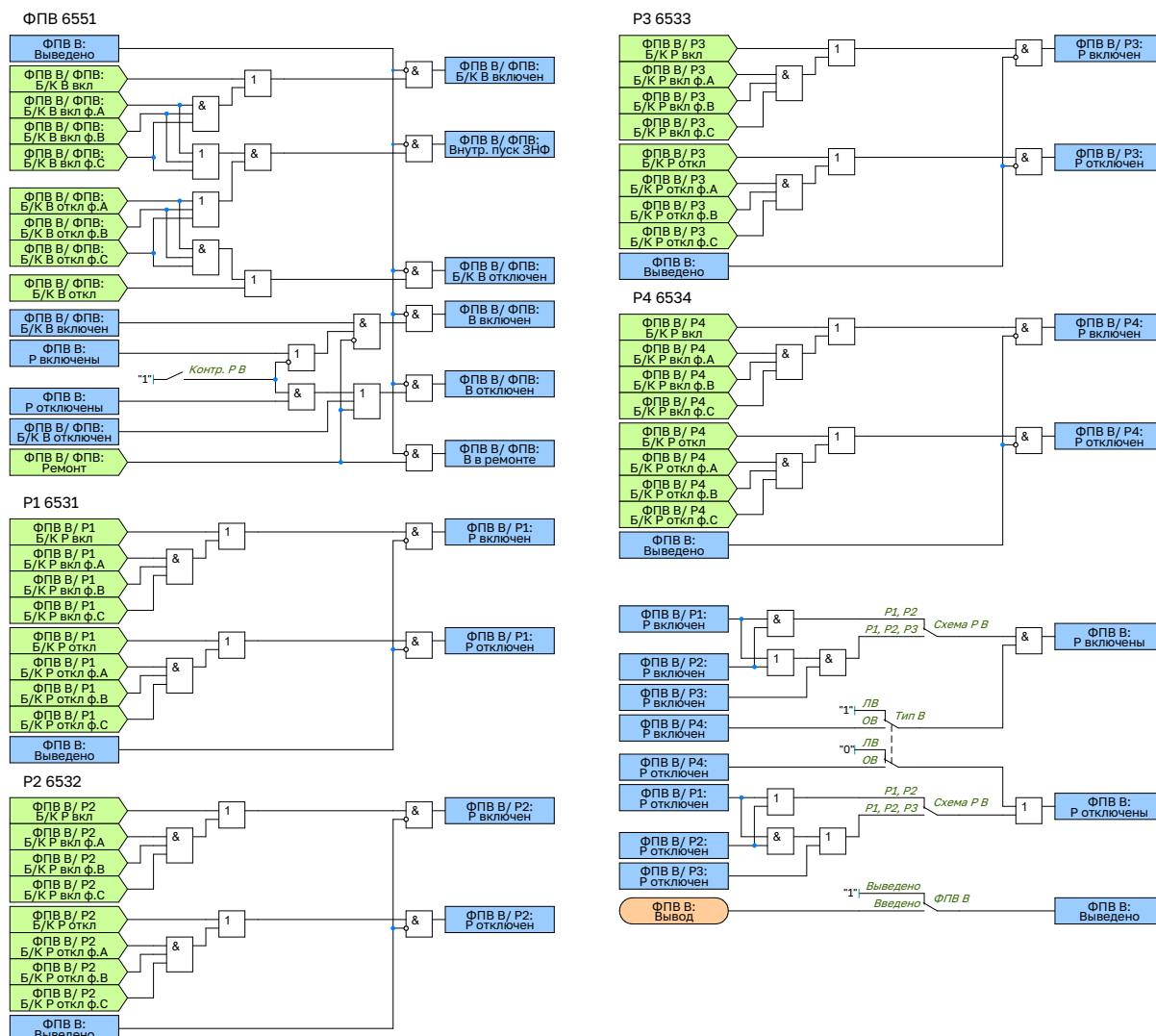
Рисунок 2.24 – Функциональная схема логики ФПВ В2
