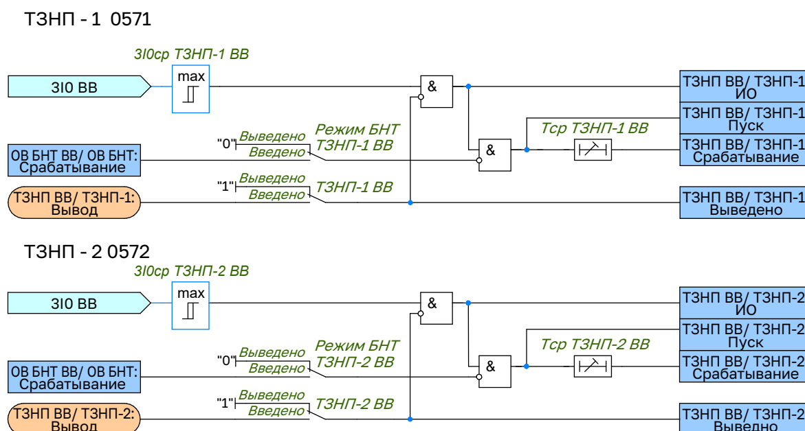
Рисунок 2.14 – Функциональная схема логики ТЗНП ВВ
